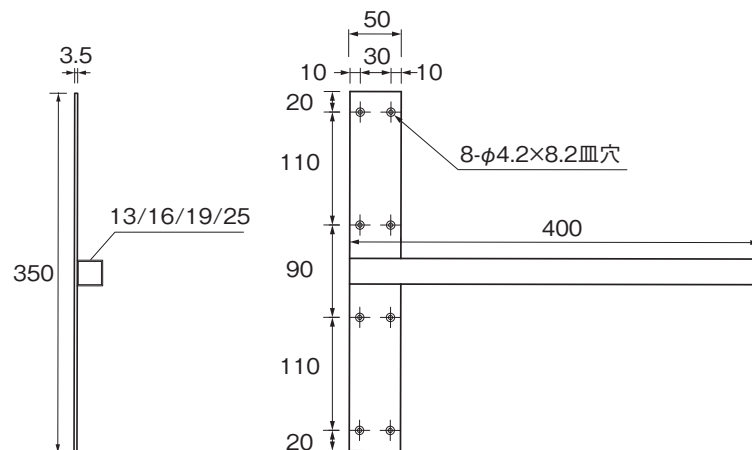
取付プレート幅50mm 寸法図
