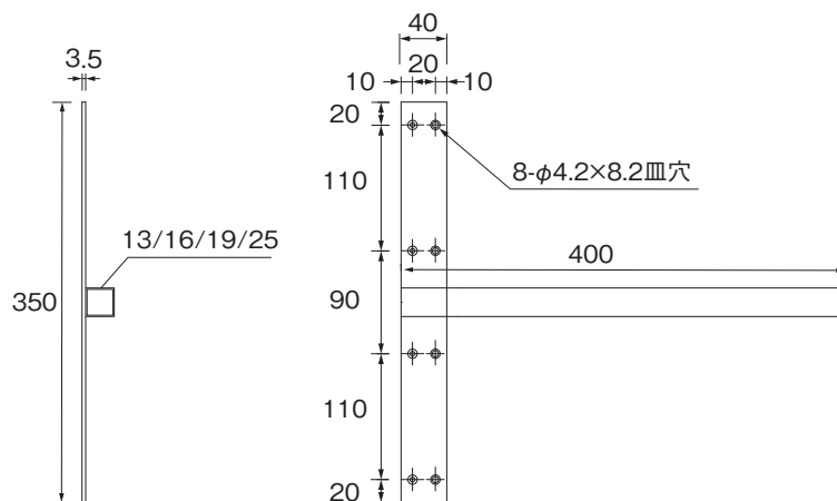
取付プレート幅40mm 寸法図
