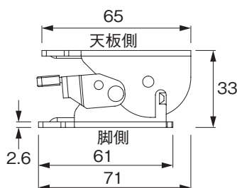
折畳時の寸法図
