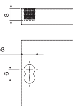
取付穴加工図
