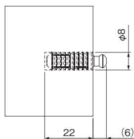
取付穴加工図
