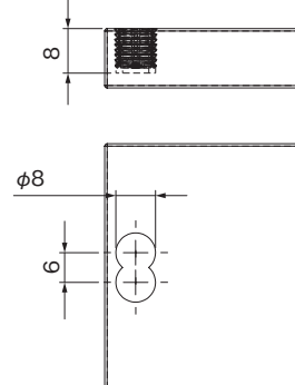
取付穴加工図
